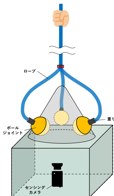
図3：髪の毛型ロープデバイス構造
