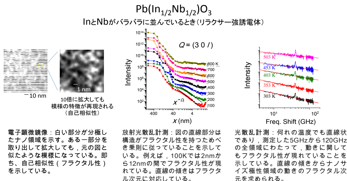
図 2. \text{Pb}(\text{In}_{1/2}\text{Nb}_{1/2})\text{O}_3 において In 原子と Nb 原子がバラバラに並んでいるとき(リラクサー強誘電体)の実験結果。(左)電子顕微鏡像。(中)放射光 X 線散乱計測。(右)光散乱計測。
