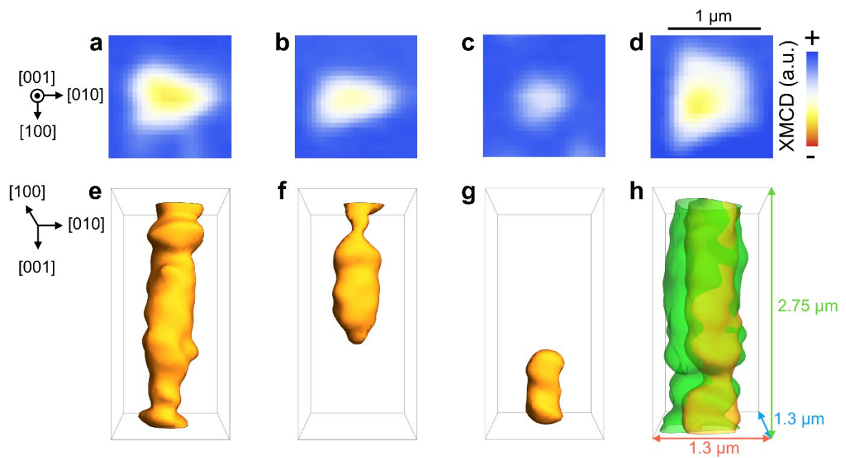
図3：(a)-(d)個々のスキルミオンひもを真上から観察した際の二次元 XMCD 透過像。(e)-(h) それぞれに対応する、トモグラフィー測定によって得られたスキルミオンひもの三次元形状。スキルミオンひもは概ね真っ直ぐな形状をしているが、結晶中の欠陥の影響などを反映して、複雑な凹凸を有していることが読み取れる。(e),(h)では試料の中をスキルミオンひもが貫通しているのに対して、(f),(g)では途中でひもが切れている。(h)における緑色のデータは、[001] 方向に加えている外部磁場の値を小さくした場合の形状変化を表している。
