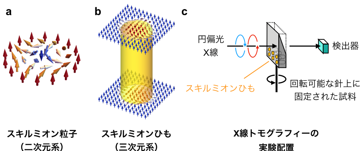
図 1：(a)二次元系におけるスキルミオン粒子の模式図。矢印はスピンの向きを示している。(b)三次元系におけるスキルミオンひもの模式図。二次元的なスキルミオンが、ひも方向に一樣に積層した構造を有している。(c)本研究における X 線トモグラフィ実験の測定配置。さまざまな角度から観察した二次元 XMCD 透過像をもとに、図 2・図 3 に示すようなスキルミオンひもの三次元形状の再構築を行った。
