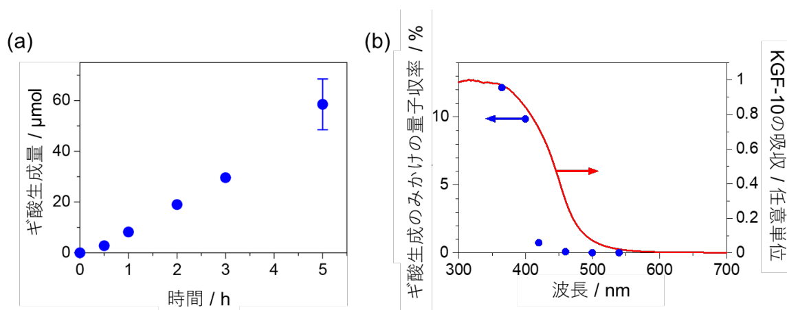
図 3. (a) ギ酸生成の時間経過。種々の実験により、初めの 30 分程度で構造が変化してから直線的にギ酸が生成していることから、光触媒反応と確認された。(b) KGF-10 の吸収とみかけの量子収率の作用スペクトル（用語 5）。KGF-10 の吸収（赤線）が 530 nm 付近から急激に立ち上がっているのに対して、ギ酸生成のみかけの量子収率（青点）も同様に 540 nm からその値が立ち上がっており、KGF-10 が吸収した光エネルギーが光触媒反応に利用されていることを示している。
