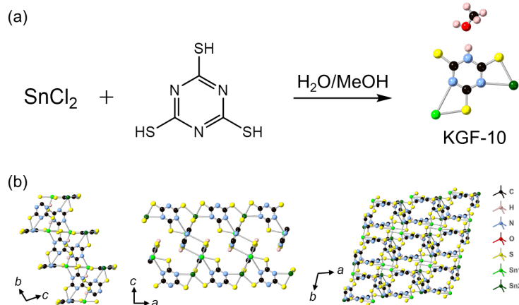
図 2. 本研究で注目した KGF-10 の (a) 反応スキームと (b) 結晶構造
