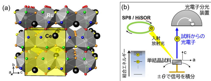
図 1 \text{CeRu}_2\text{Al}_{10} の結晶構造、ARPES 実験のセットアップ
