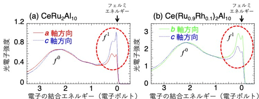
図2 CeRu 2 Al 10 と Ce(Ru 0.9 Rh 0.1 ) 2 Al 10 の実験結果
